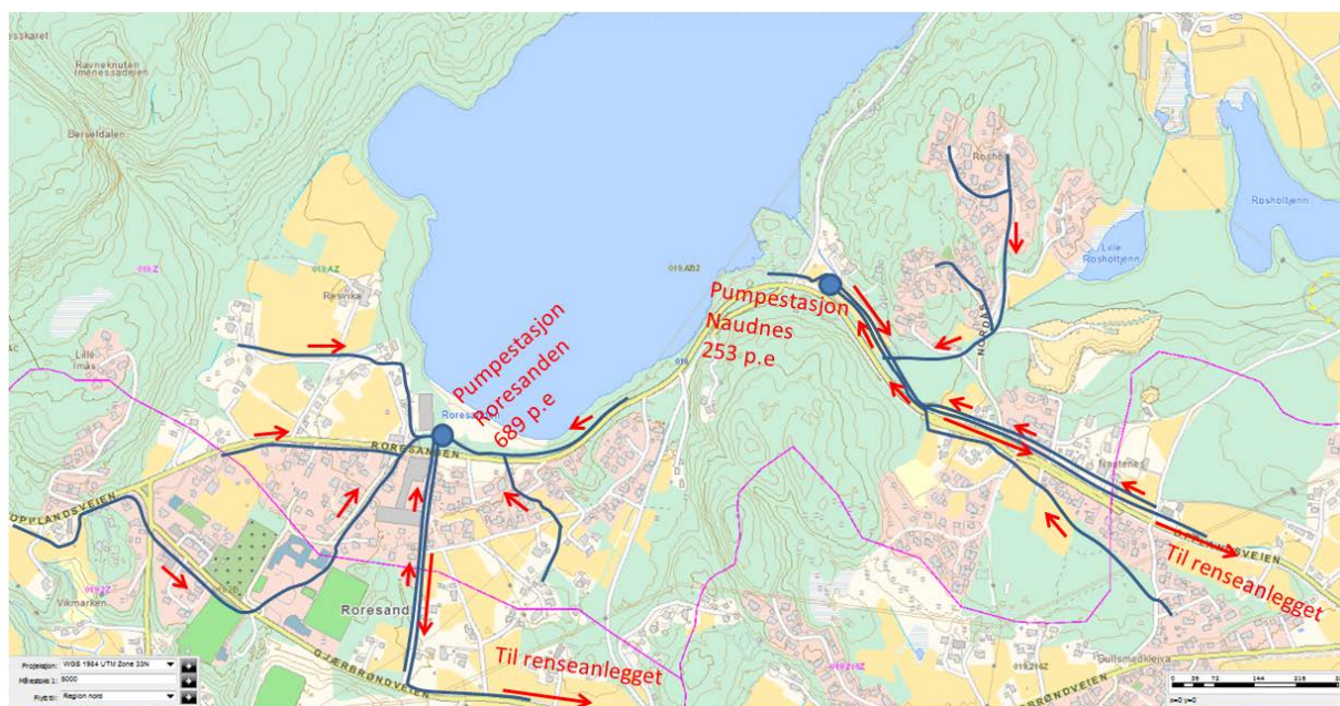
Figur 2.4. Kommunale kloakkledninger (NB samleledninger - stikkledninger ikke vist) og pumpestasjoner innenfor nedbørfeltet i søndre del av Rore. Korte røde piler er selvfallsledninger inn mot pumpestasjonene, mens lange piler er pumpeledninger ut av feltet mot renseanlegget. Nedbørfeltgrensen er tegnet inn med rosa strek. Kartgrunnlag: NVE-Atlas.
