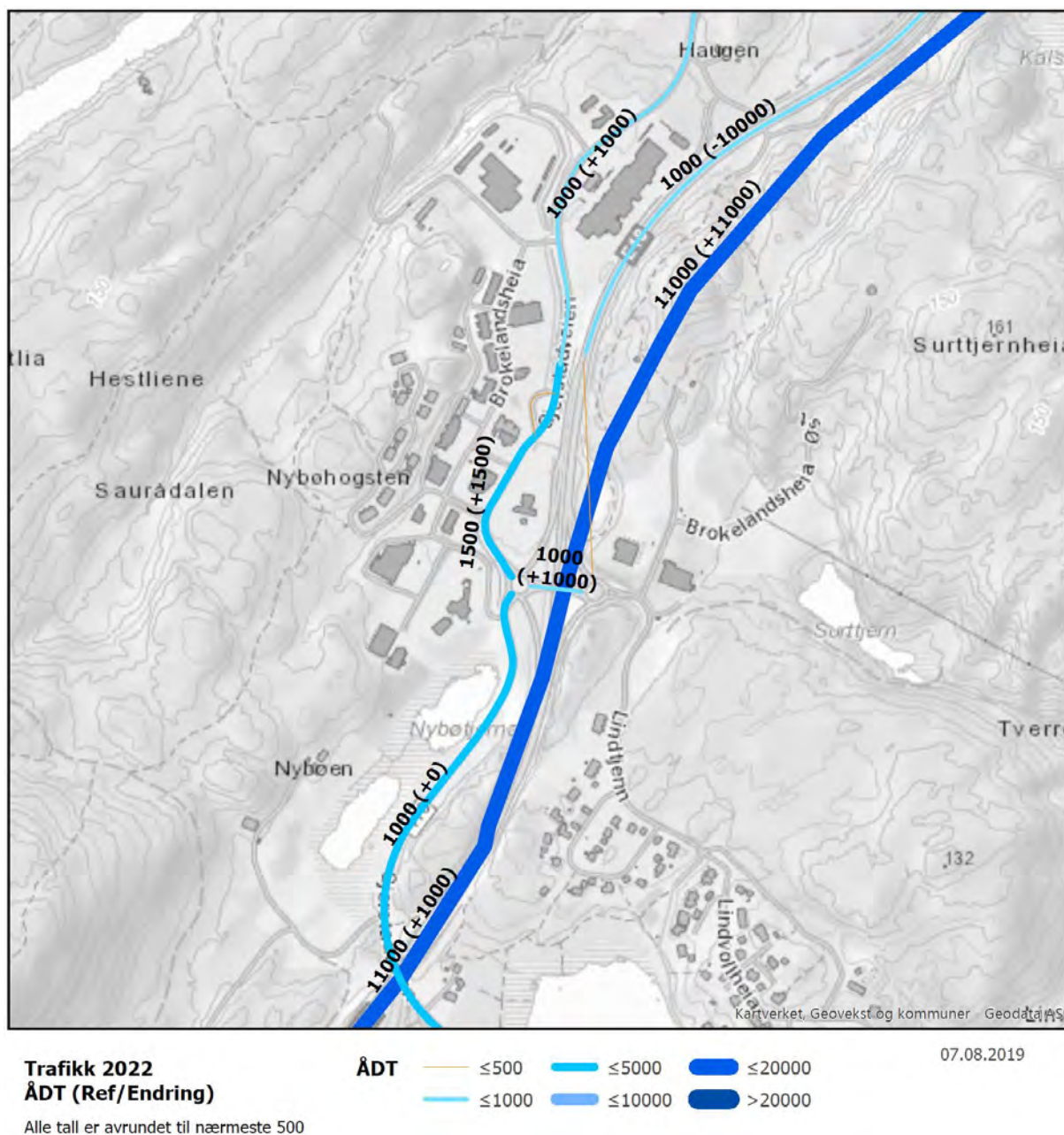
Figur 7-19 Kartet viser endring i trafikkmengde ved Brokelandsheia ved etablering av ny E18, beregnet i 2022.
