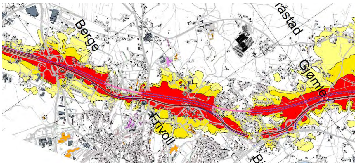
Figur 8-38 Beregnet utendørs støy fra ny E18 (tykk blå linje) uten støytiltak, med trafikkmengder for år 2060 på strekningen Gjømlen-Frivoll-Berge. Rød sone er støy over 65 dB, mørk gul sone er støy over 60 dB og lys gul sone er støy over 55 dB. Støykartet viser dagløsning for E18 gjennom Frivoldalen (høringsforslaget).
