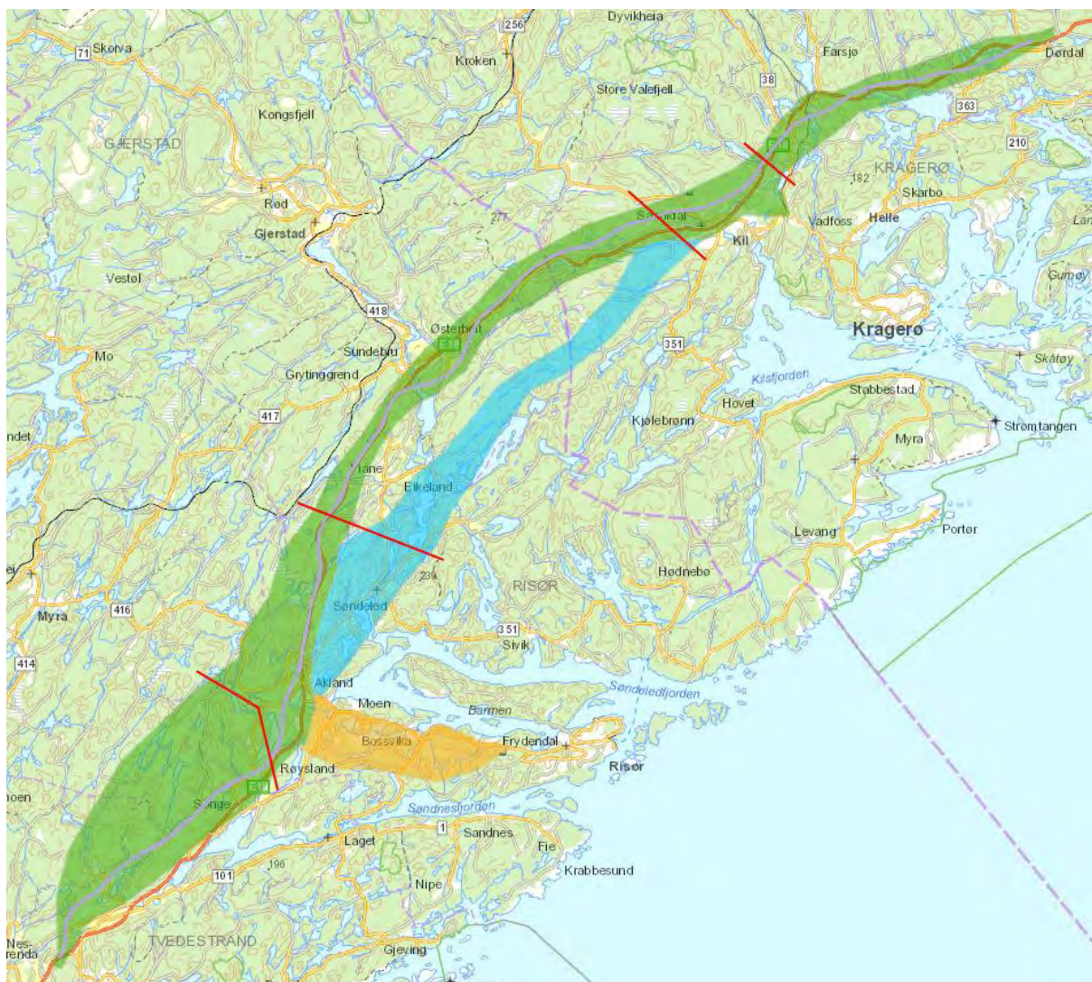
Figur 8 Veillinje 13330: 1A + 2B + 3B + 4H + 5E, vist som lilla linje
