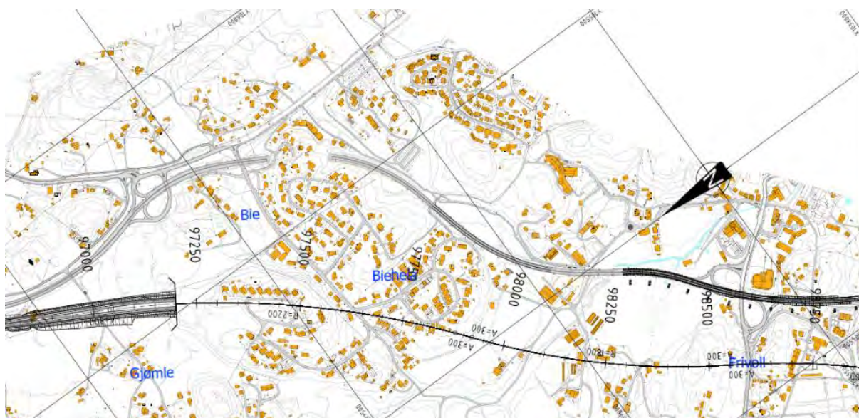
7-13 Eksempellinja går nord for dagens E18 under Frivollaldalen. Dagens kryss ved Bie, Frivoll og Øygardsdalen stenges for trafikk på E18, krysset ved Morholt opprettholdes.
