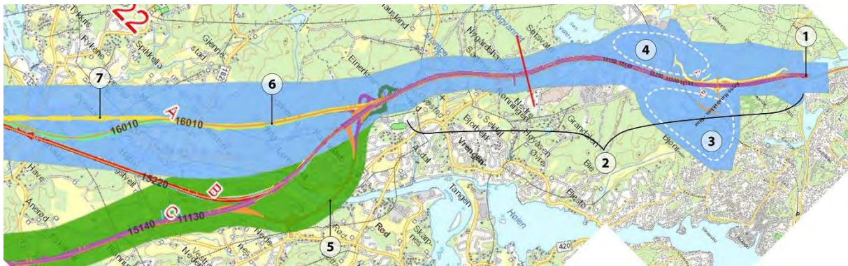
Figur 6-13: Veilinjrer innenfor planområdet i Arendal som er vurdert.
