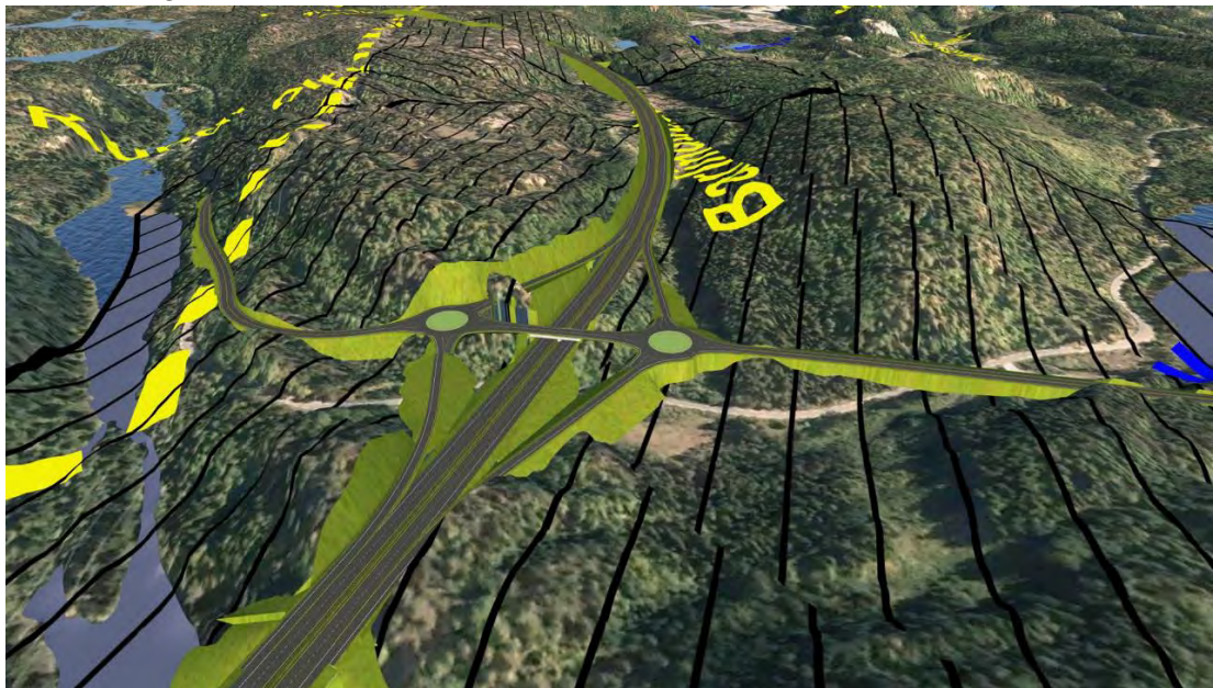
Figur 7-16 Utsnitt fra 3D-modellen som viser eksempel på plassering av Risørkryss ved Barlinddalen.
